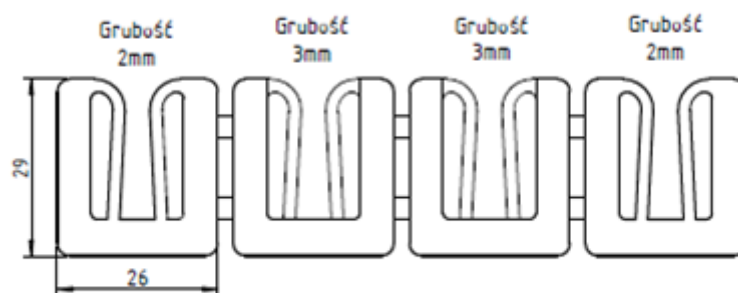
Rys.23 - zestaw podkładek dystansowych
