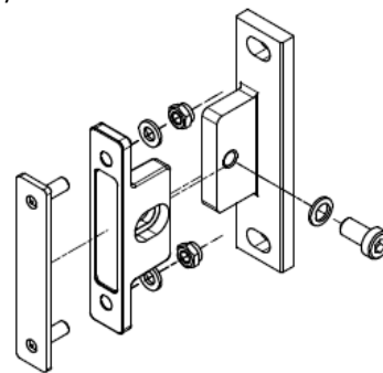
Rys. 1 Uchwyt
