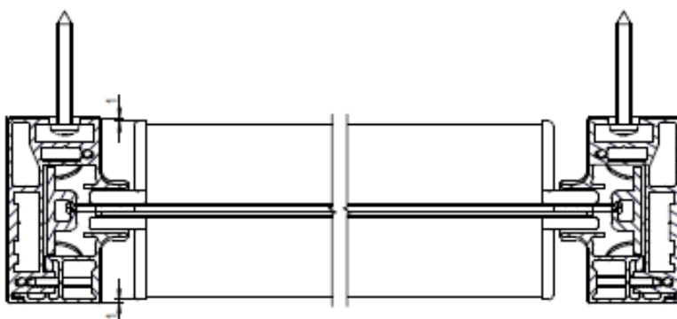
Montaż prowadnic bez użycia uchwytów (system ZIIIP120)
