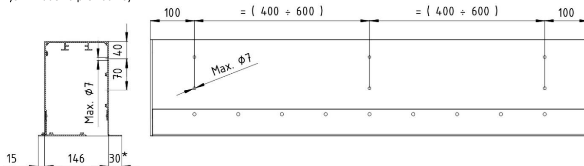
Rys. 8. Schemat wykonywania otworów montażowych w kasie podtynkowej. * - wymiar zmienny, standardowo 30 mm.
