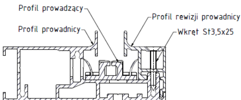
Rys. 6. Sposoby montażu prowadnicy: a) – Montaż dookienny b) – Montaż wnątkowy.
