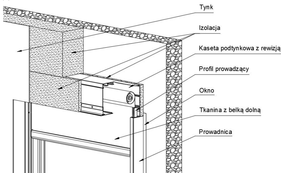
Rys. 4. Schemat Refleksol Ziiip 120 BOX - z kasetą podtynkową.
