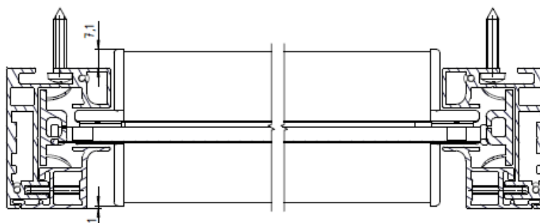
Montaż prowadnic z użyciem uchwytów (system ZIIIP120)
