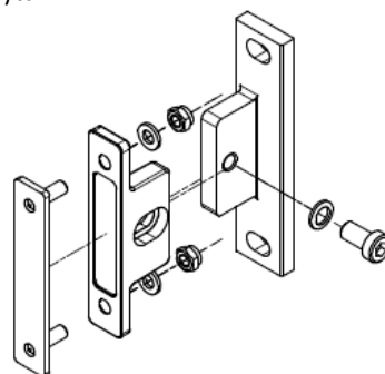
Rys. 1 Uchwyt
