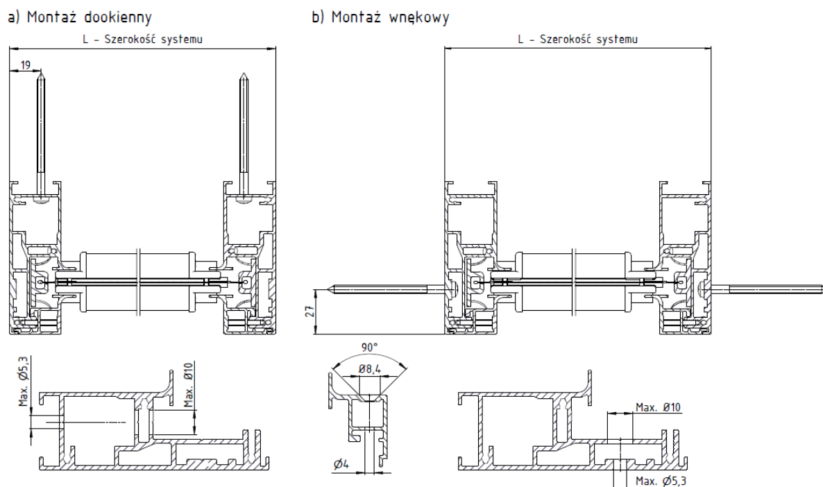
Rys. 6. Sposoby montażu prowadnicy: a) – Montaż dookienny b) – Montaż wnątkowy.
