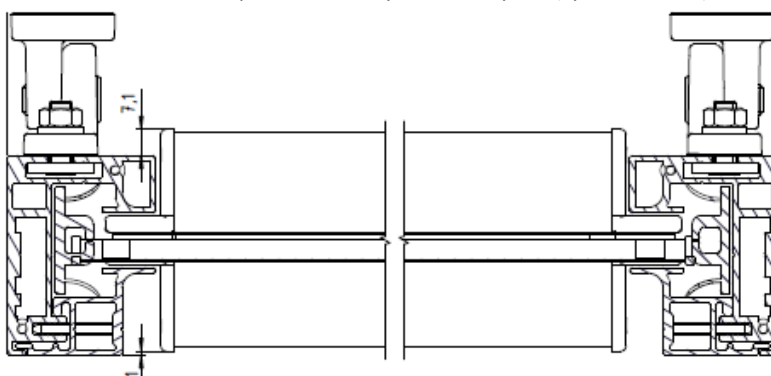
Montaż prowadnic z użyciem uchwytów (system ZIIIP95)
